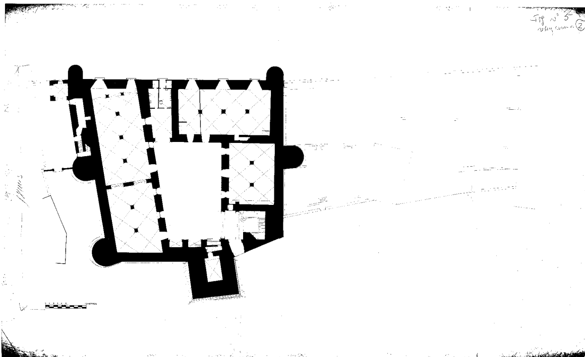
Figura 4. Planta à cota do pátio antes das obras de adaptação do castelo em pousada. Sistema de Informação para o Património Arquitectónico (SIPA.DES.00042107), Forte de Sacavém.
