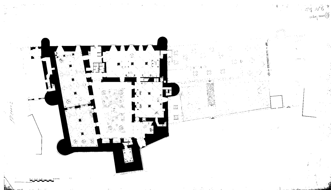
Figura 5. Planta à cota do pátio depois das obras de adaptação do castelo em pousada. Sistema de Informação para o Património Arquitectónico (SIPA.DES.00042103), Forte de Sacavém.
